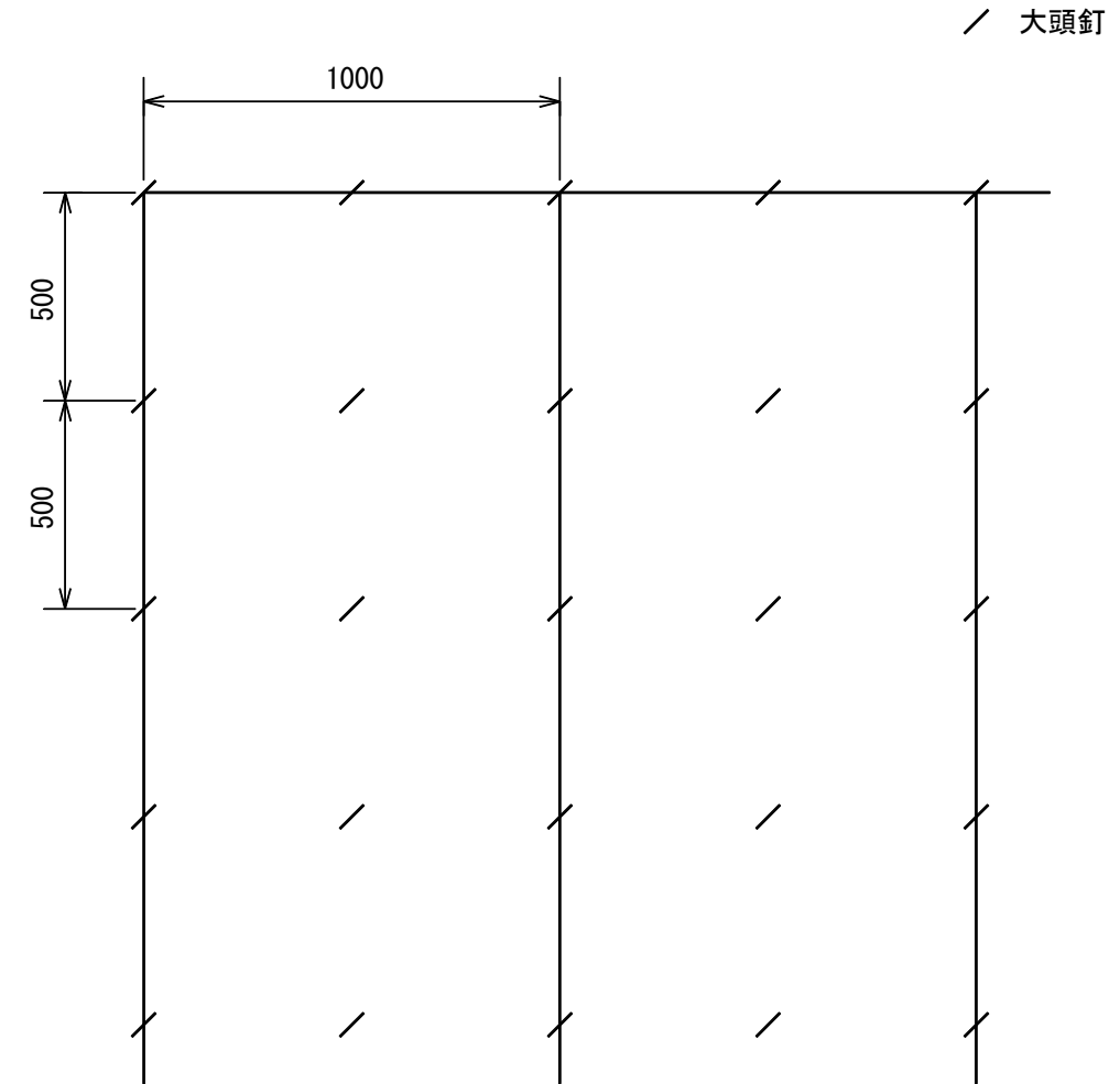
標準展開図
