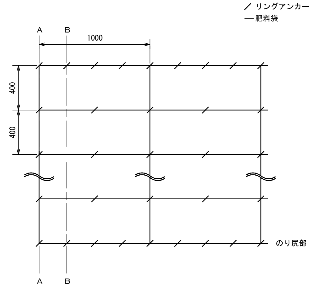
標準展開図
