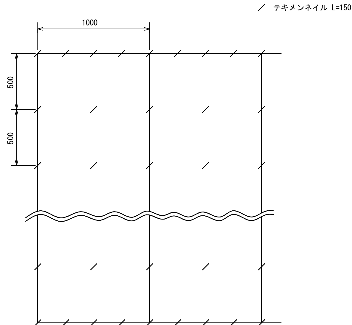
標準展開図
