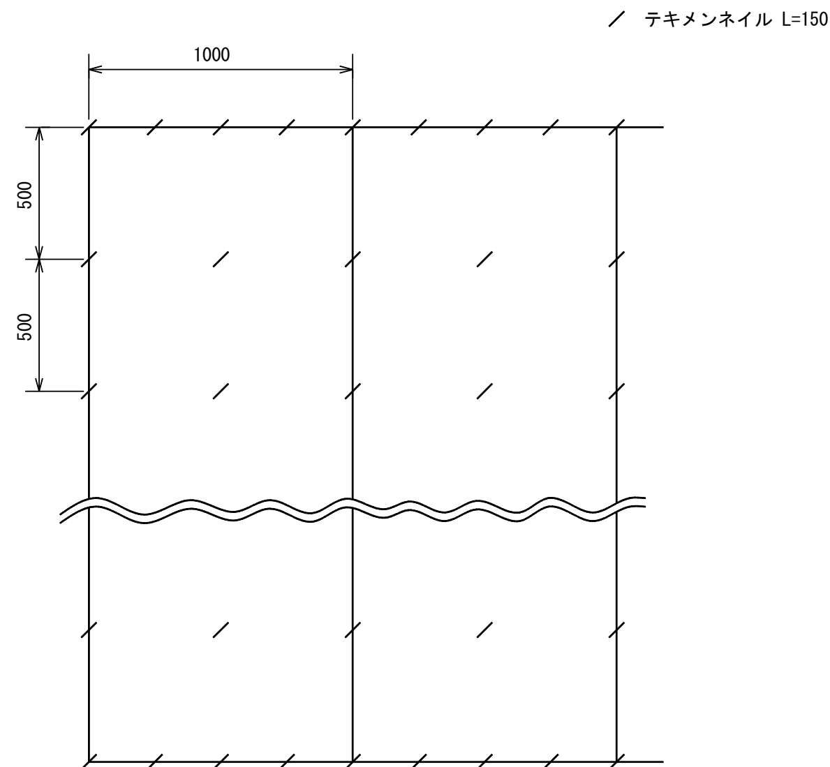
標準展開図
