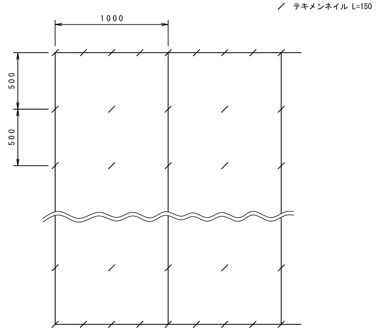
標準展開図
