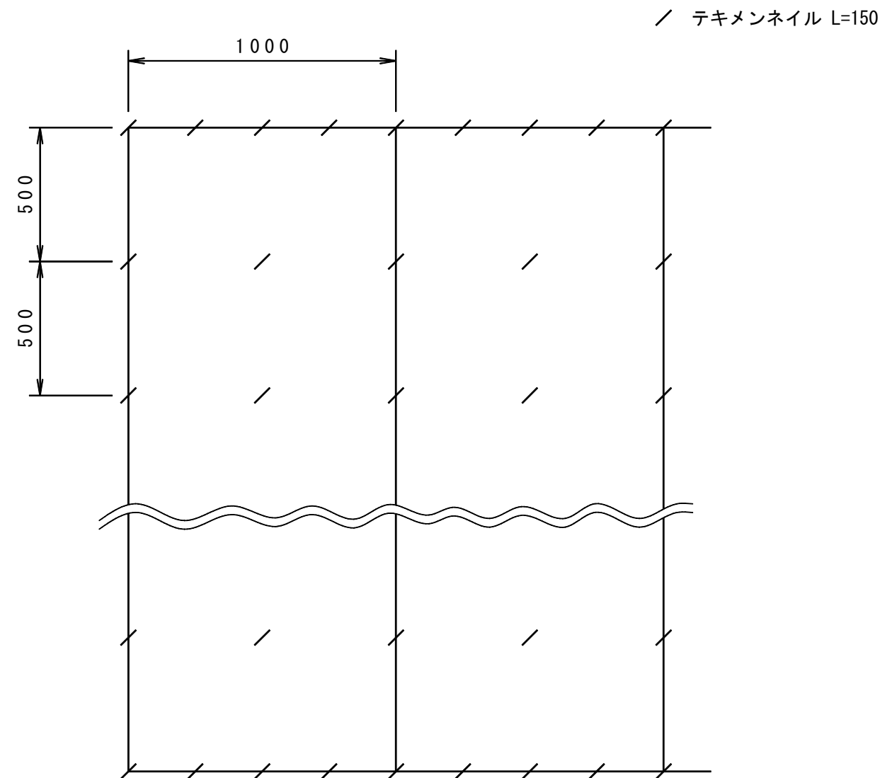
標準展開図
