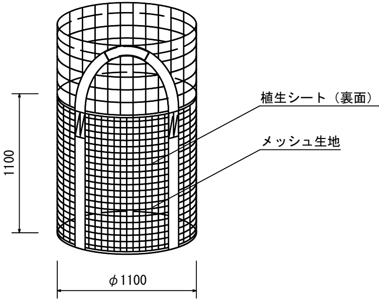
メガ・メデル構造図 (1/30)
