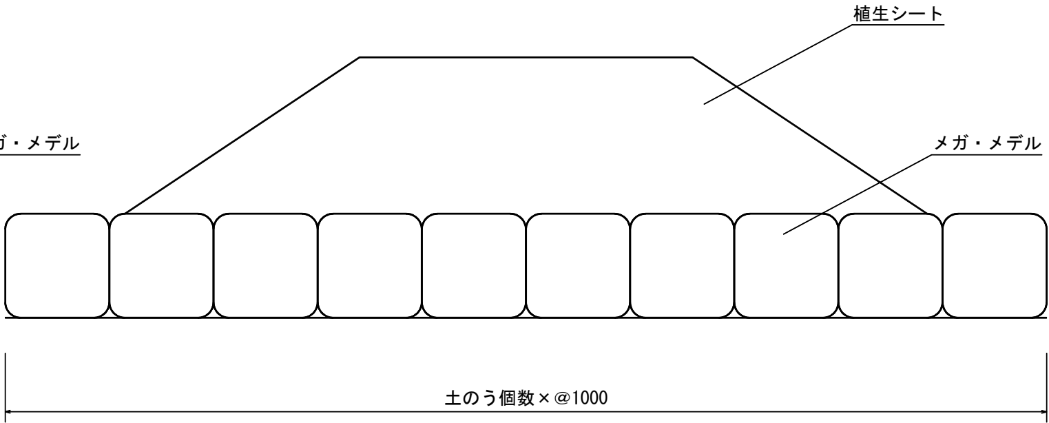
正面図
