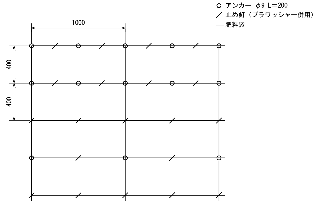
標準展開図
