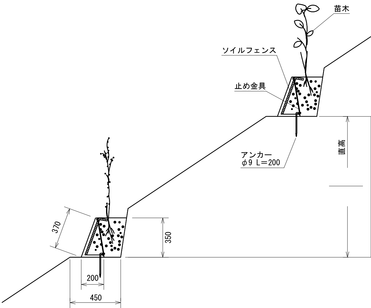
標準断面図
