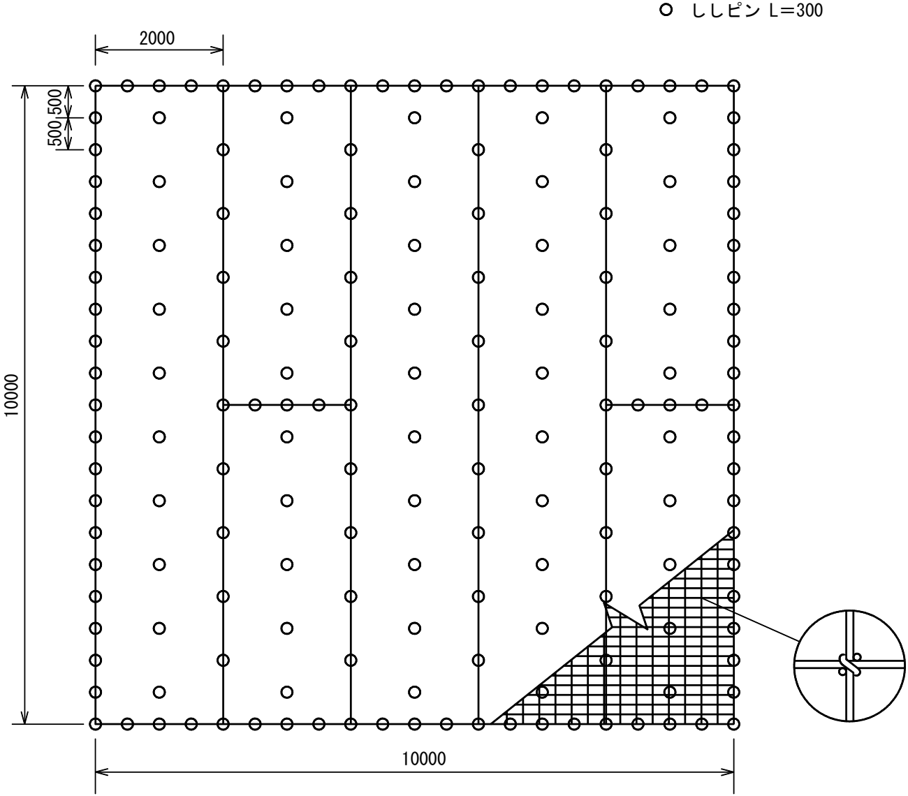
標準展開図 (S=1/80)
