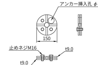
ホールドプレート 岩部交点用
