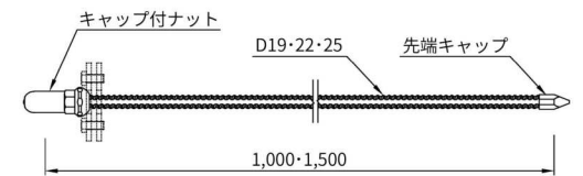
岩部用アンカー
