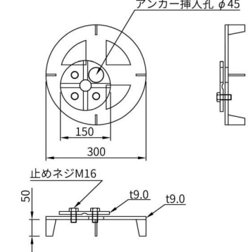
ホールドプレート 土砂部交点用
