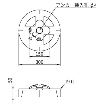
ホールドプレート 土砂部外周用
