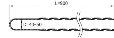
巻付グリップ
