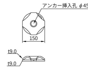
ホールドプレート 岩部外周用
