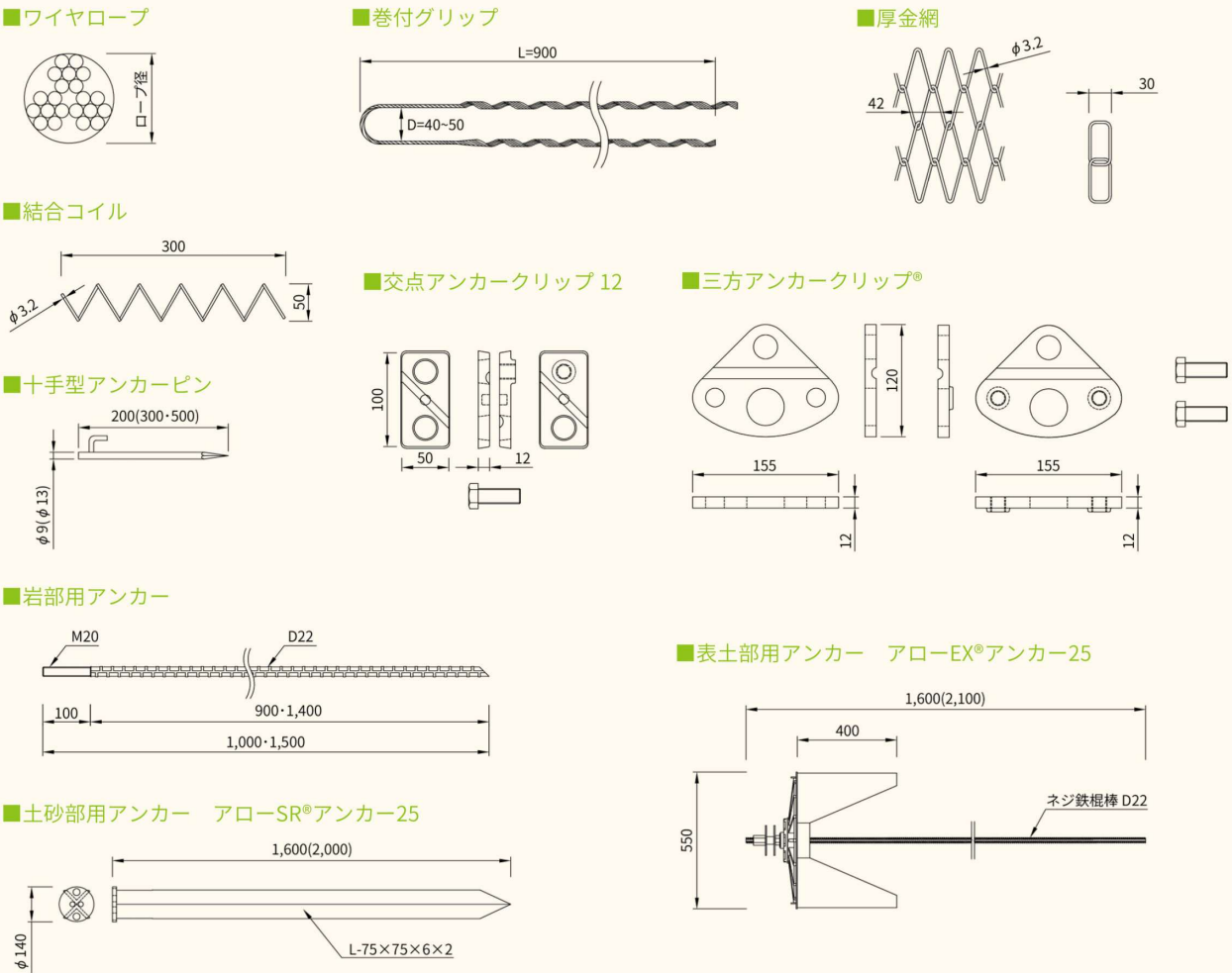
部品図
