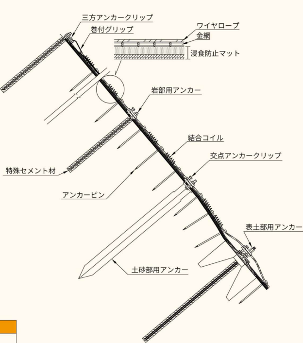
横断面図
