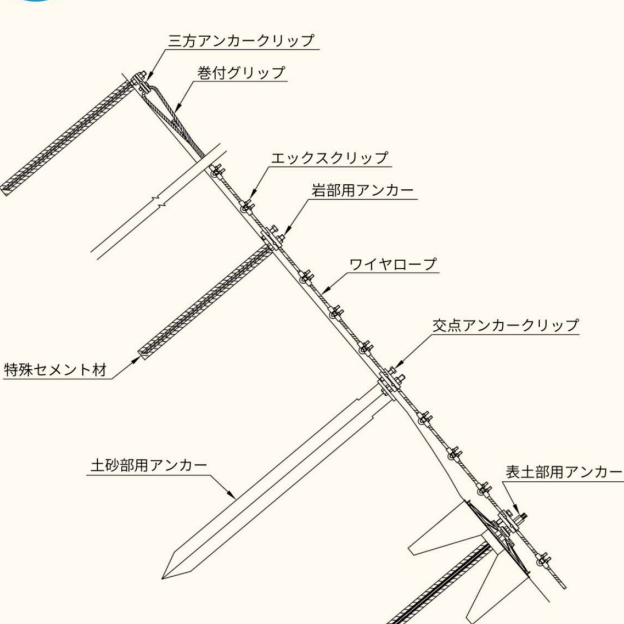
横断面図
