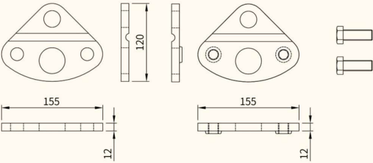
■三方アンカークリップ®
