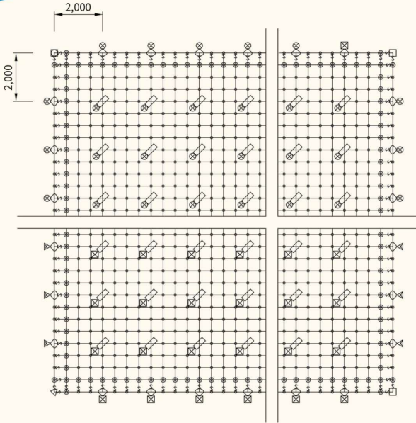
展開図
