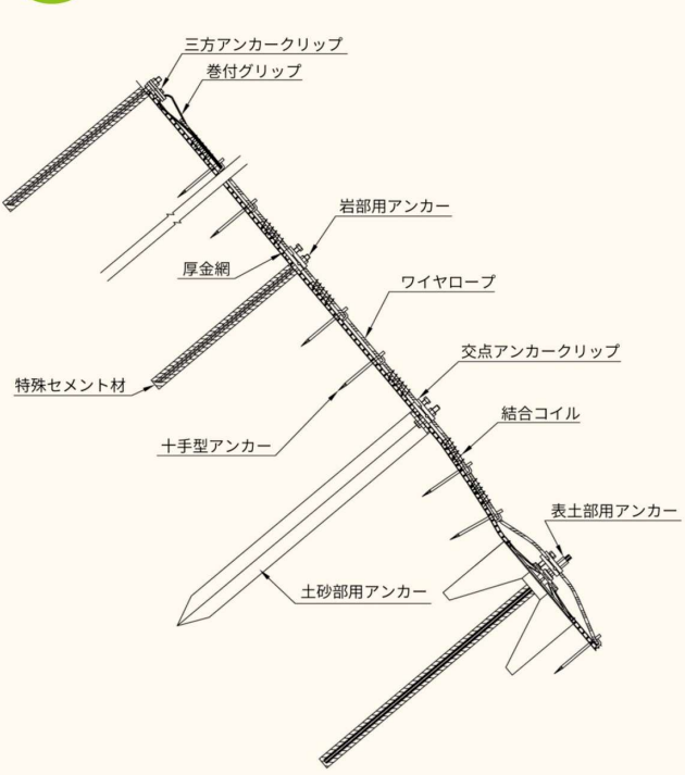
横断面図
