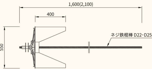
■表土部用アンカー アローEX®アンカー-25・35
