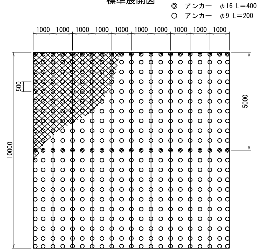
標準展開図
