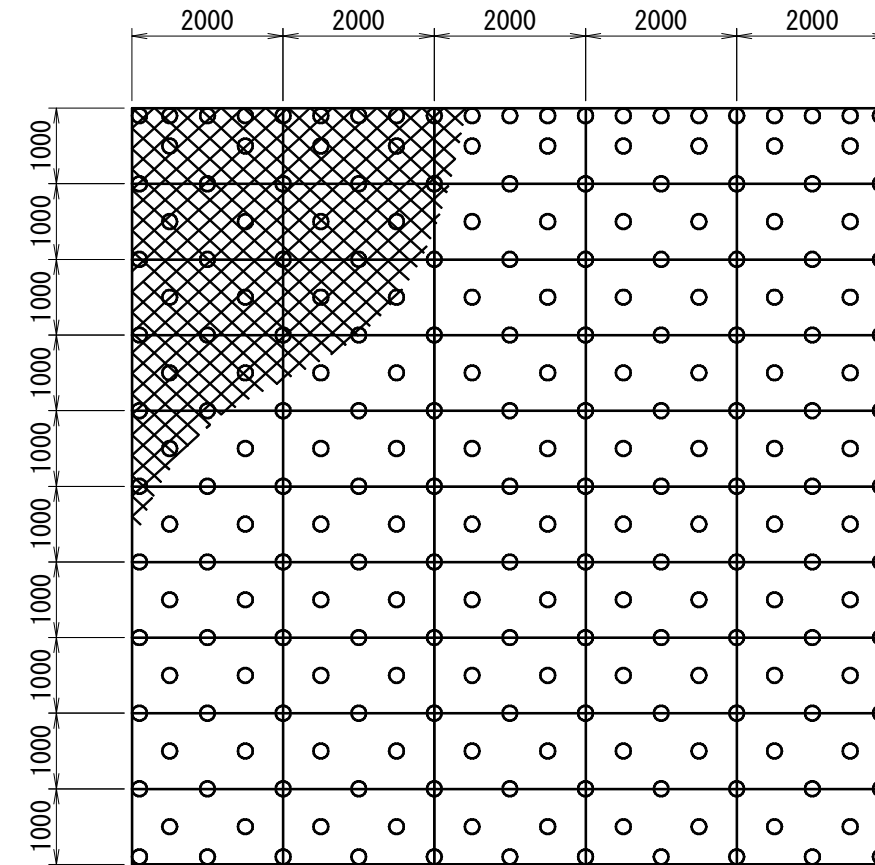
標準展開図
