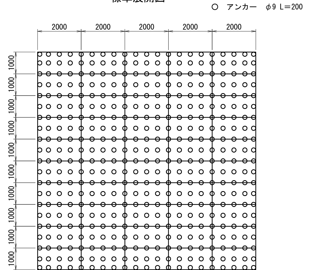
標準展開図
