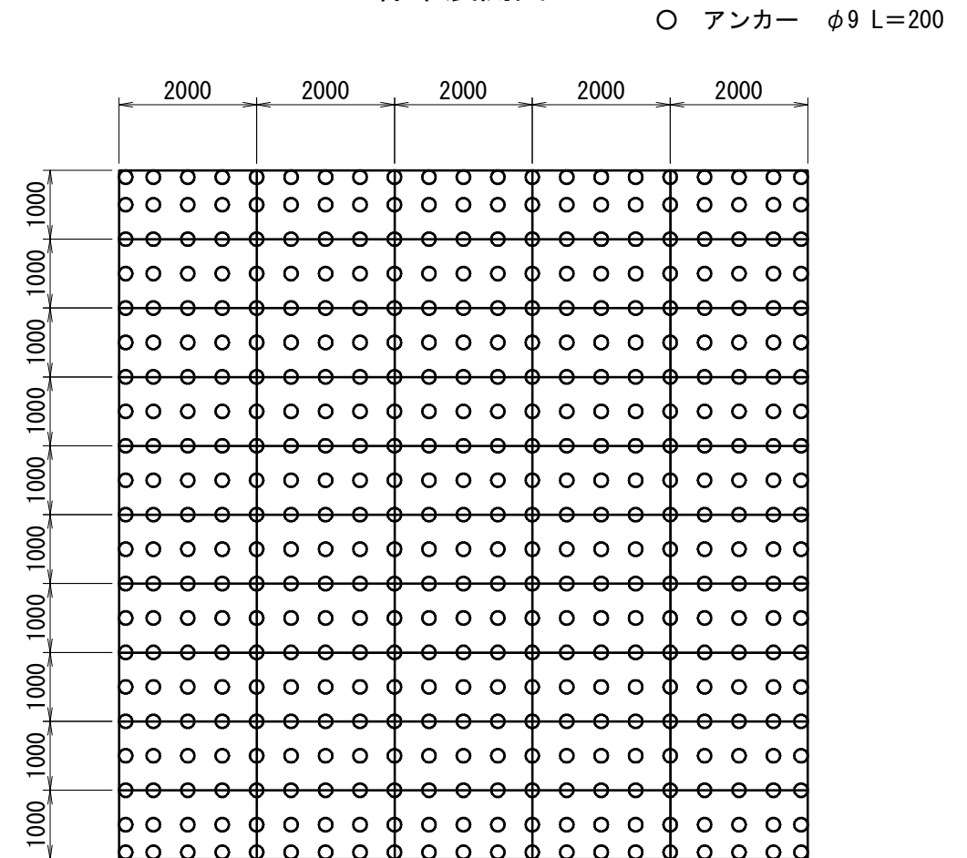
標準展開図
