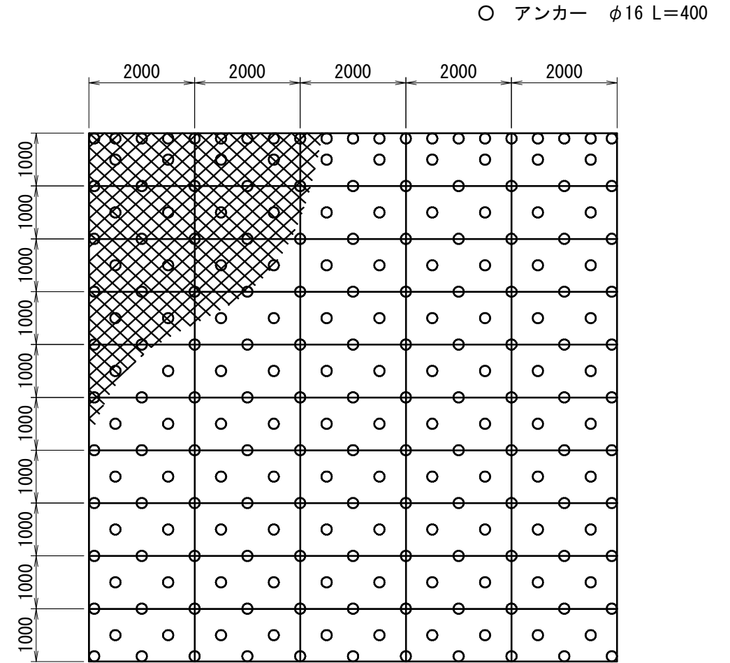
標準展開図
