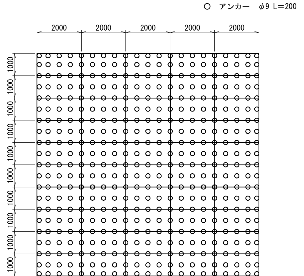
標準展開図
