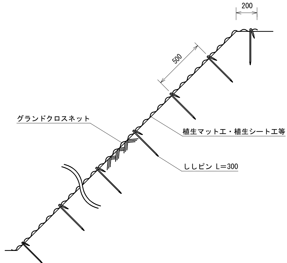
標準断面図
