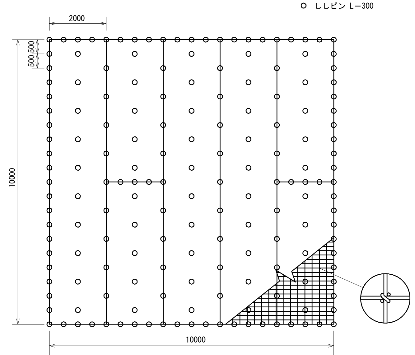
標準展開図 (S=1/80)
