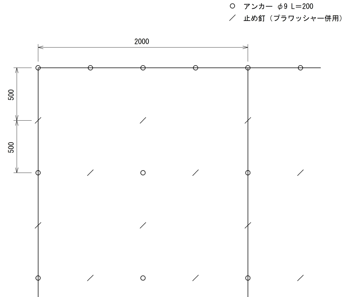
標準展開図
