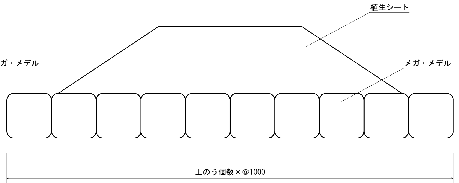
正面図
