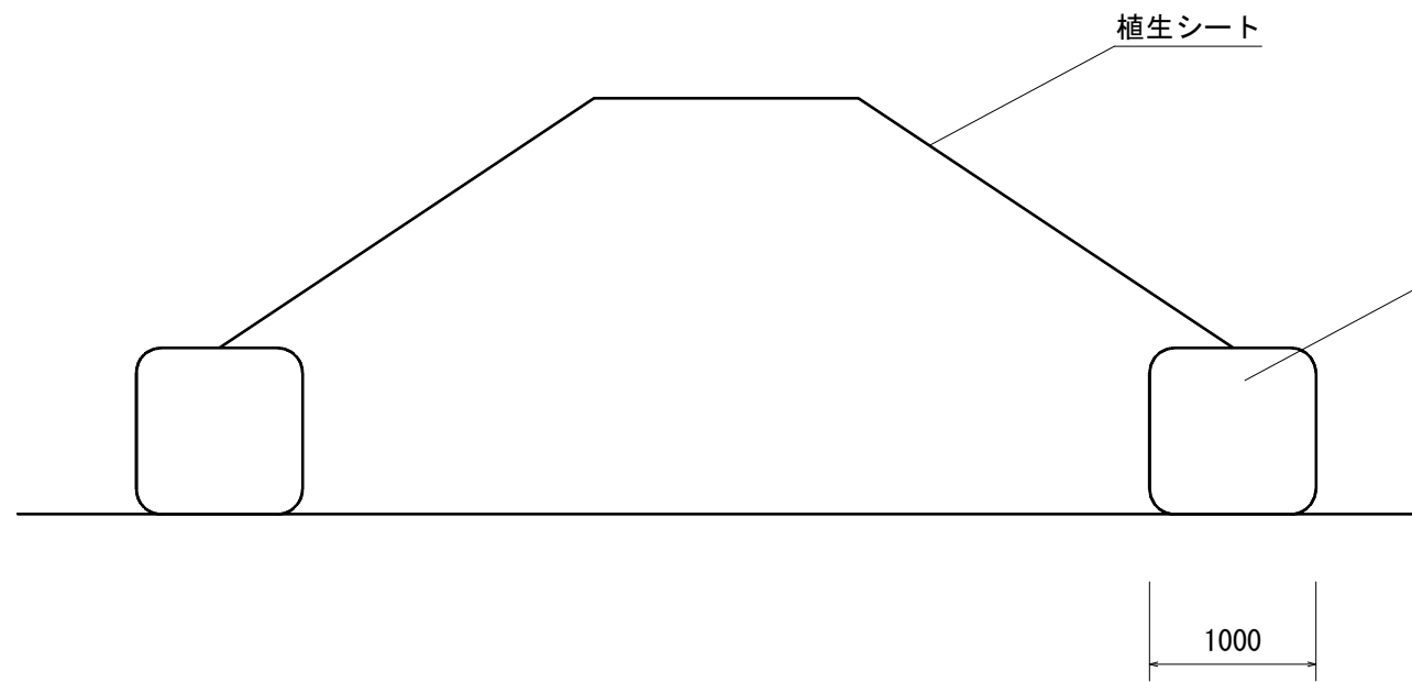
断面図
