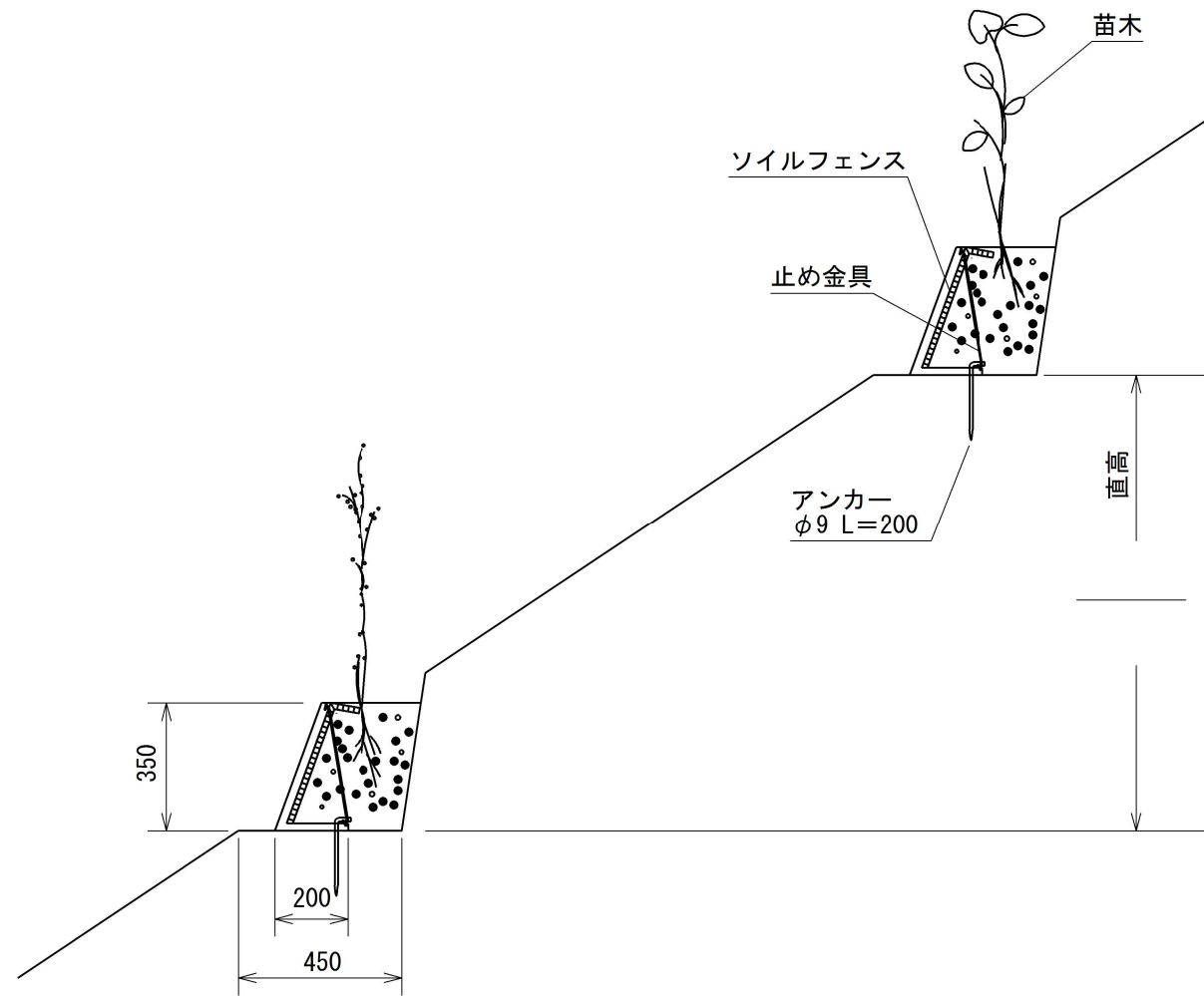
標準断面図
