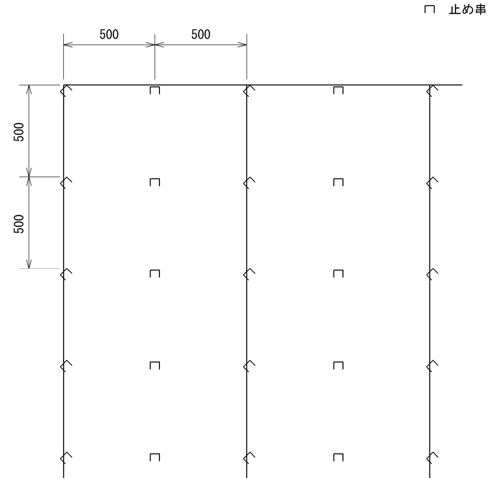
標準展開図
