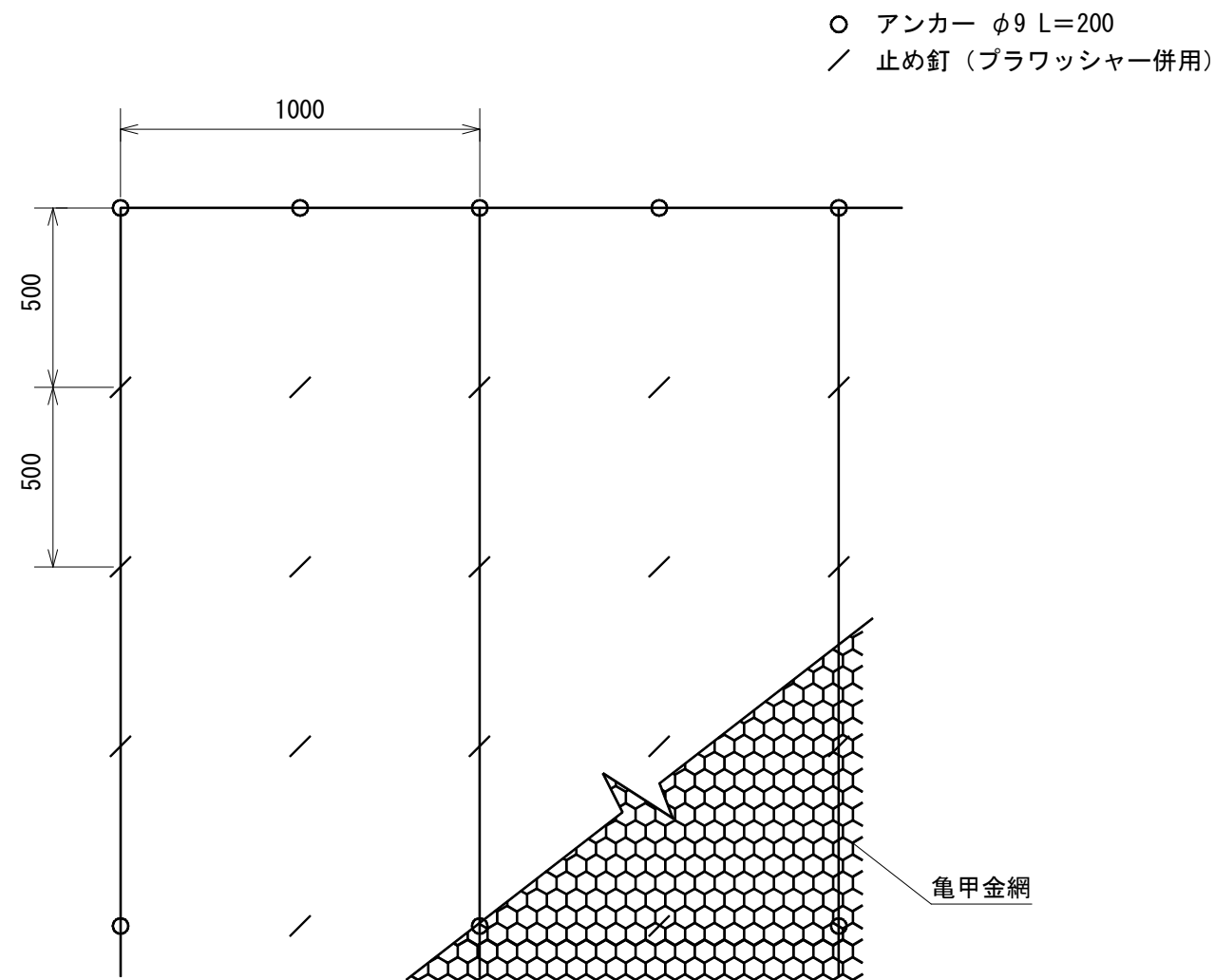
標準展開図
