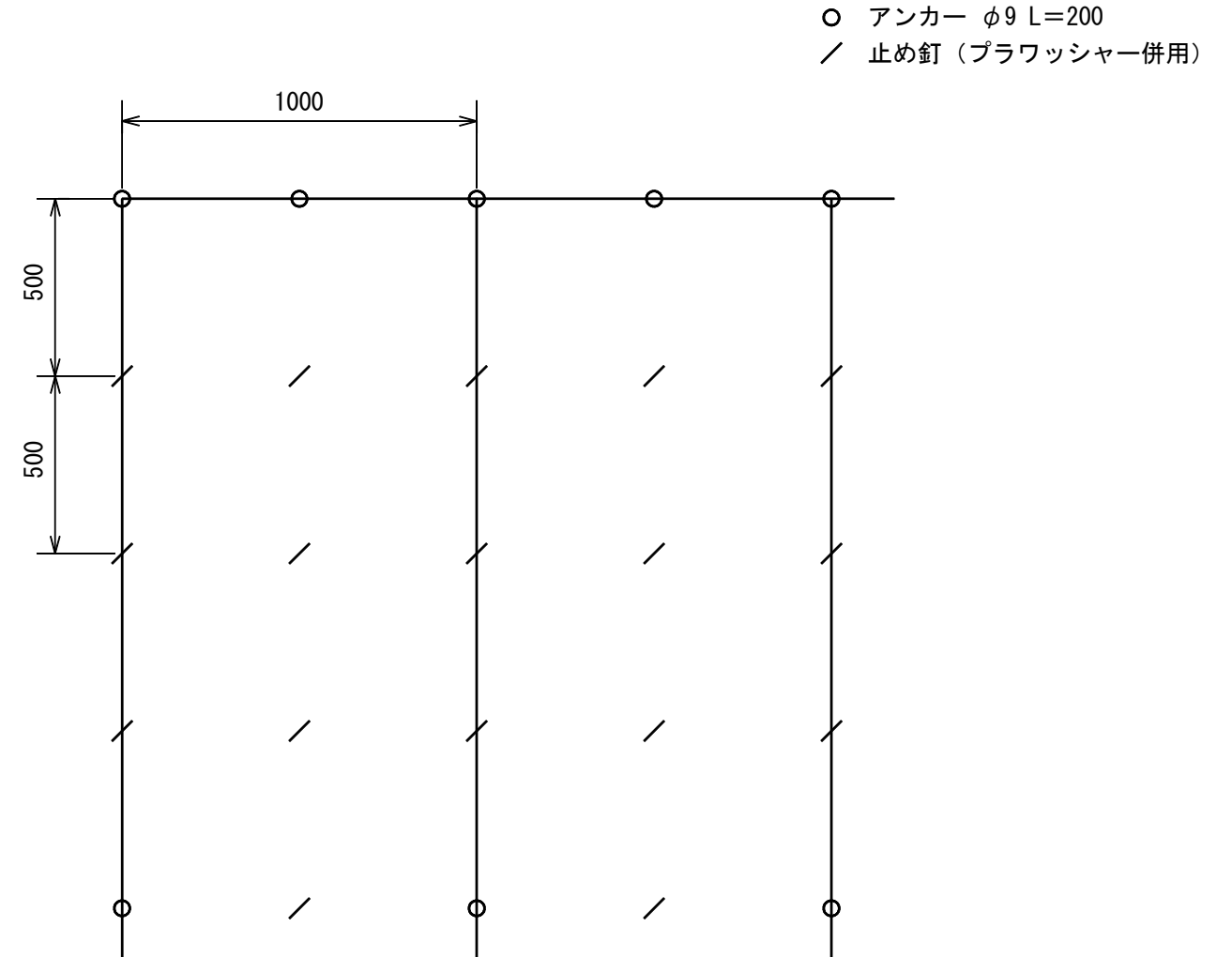
標準展開図
