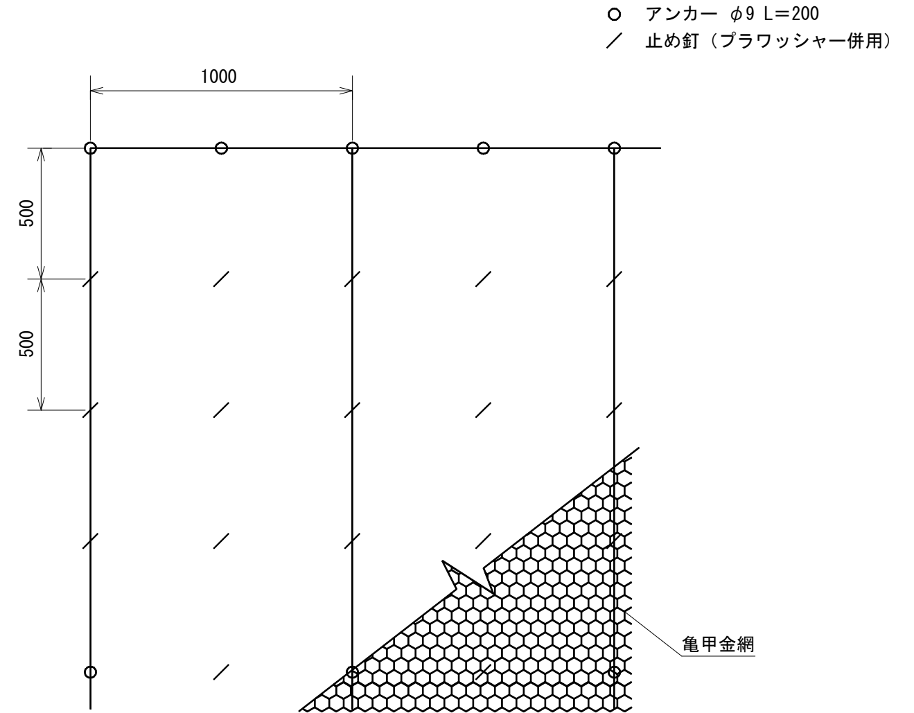
標準展開図
