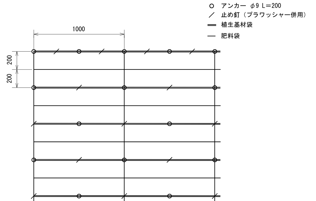
標準展開図
