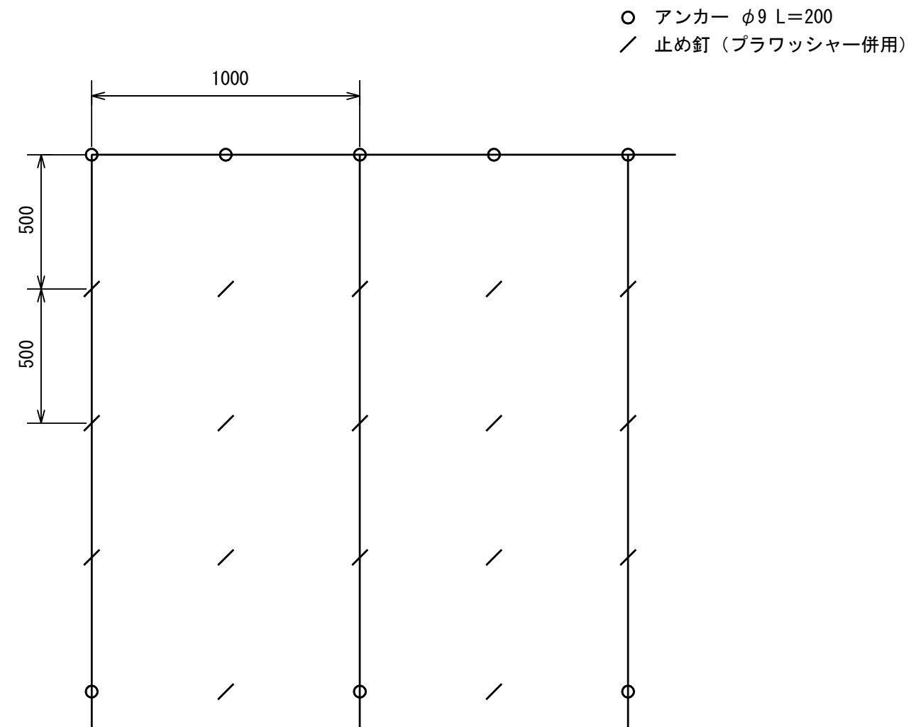
標準展開図
