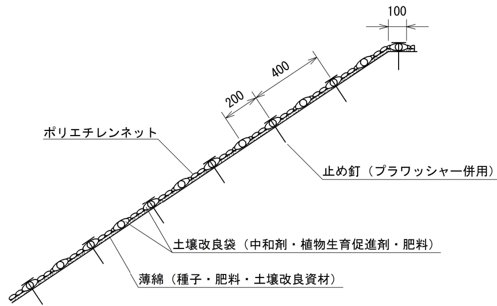
標準断面図
