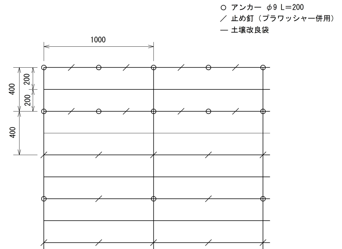
標準展開図
