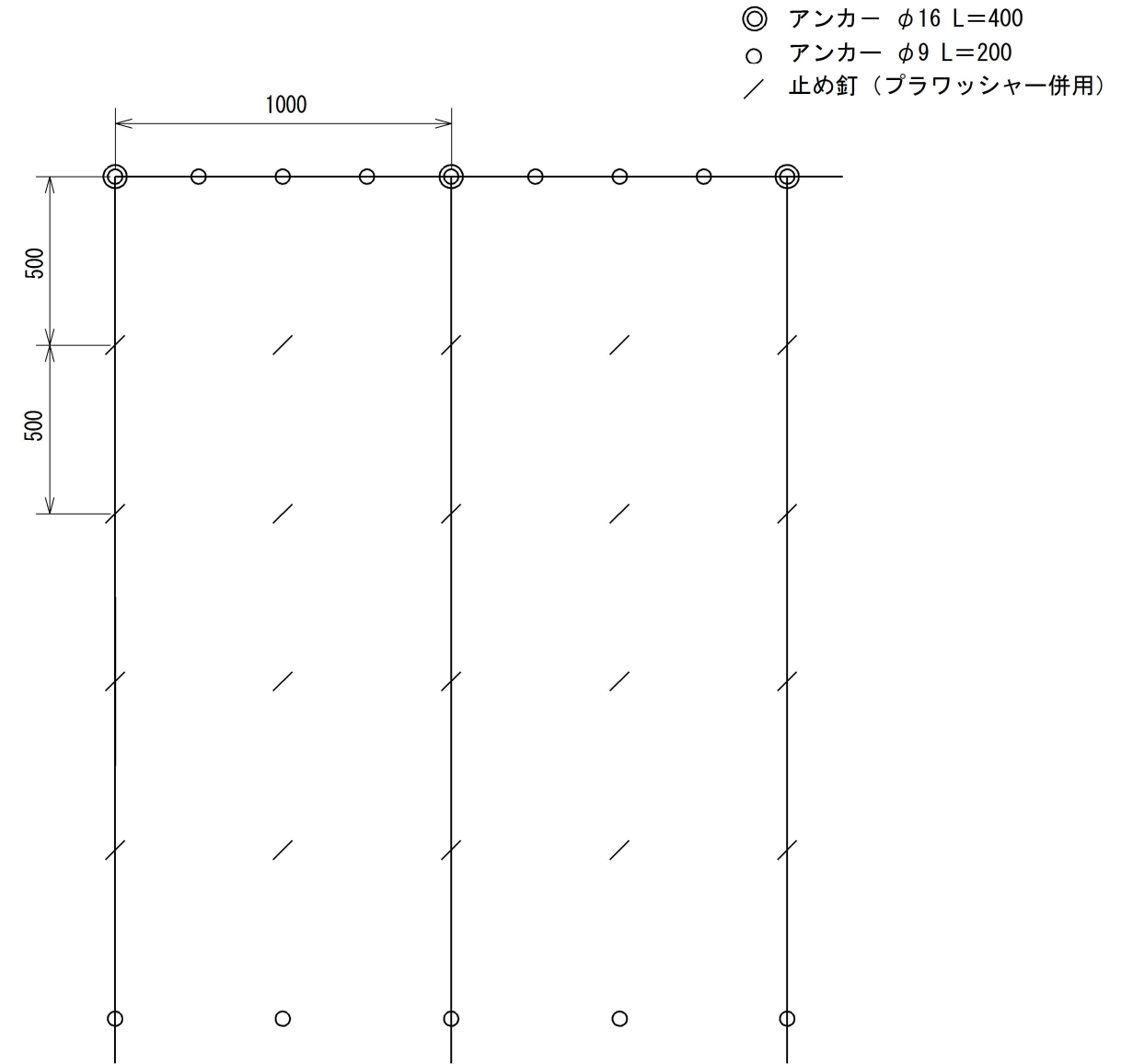
標準展開図
