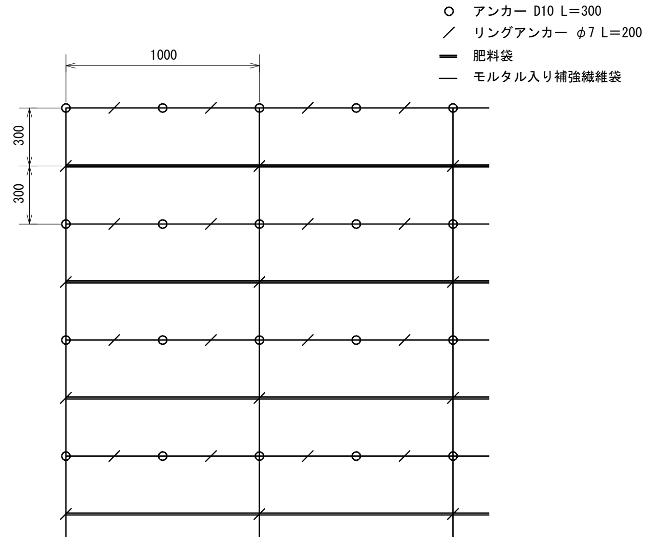
標準展開図
