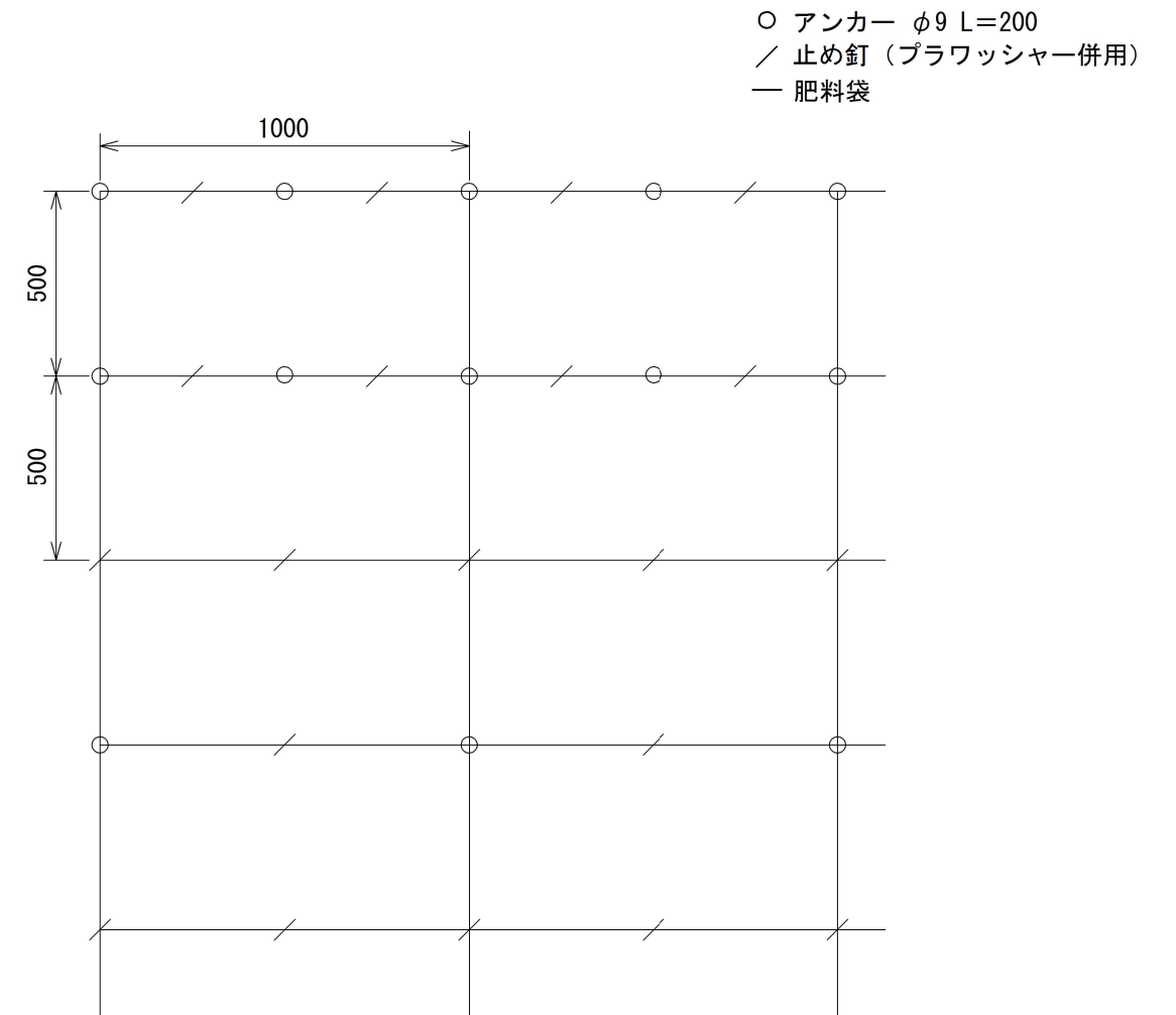
標準展開図
