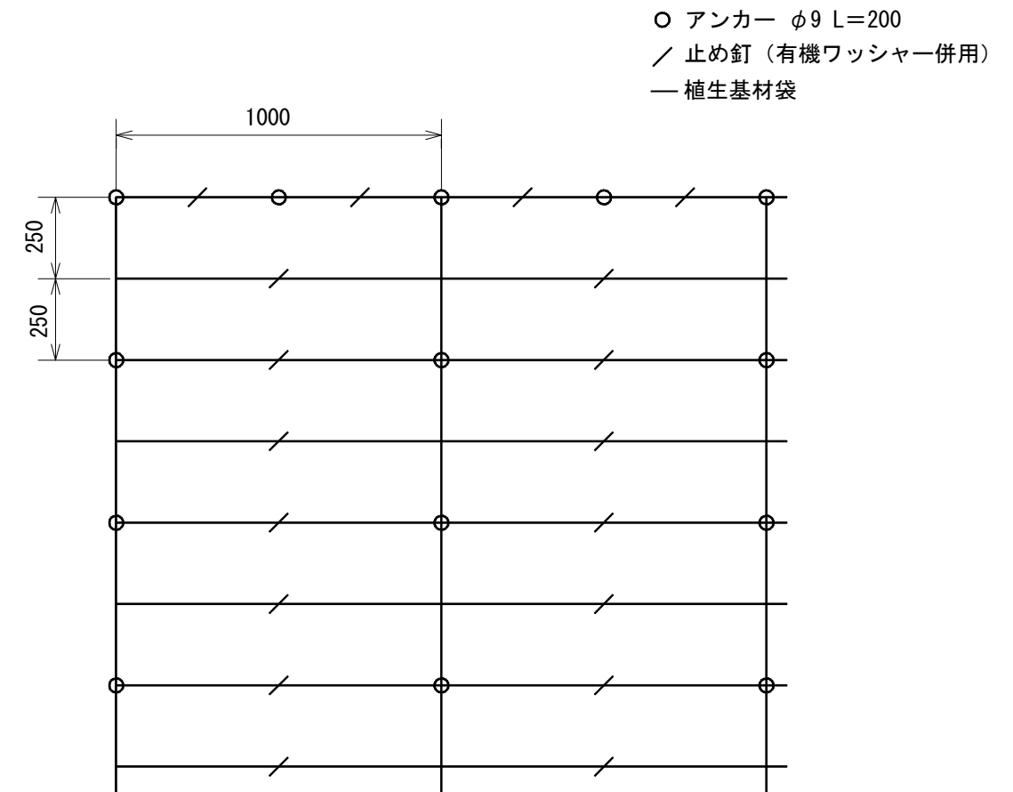
標準展開図
