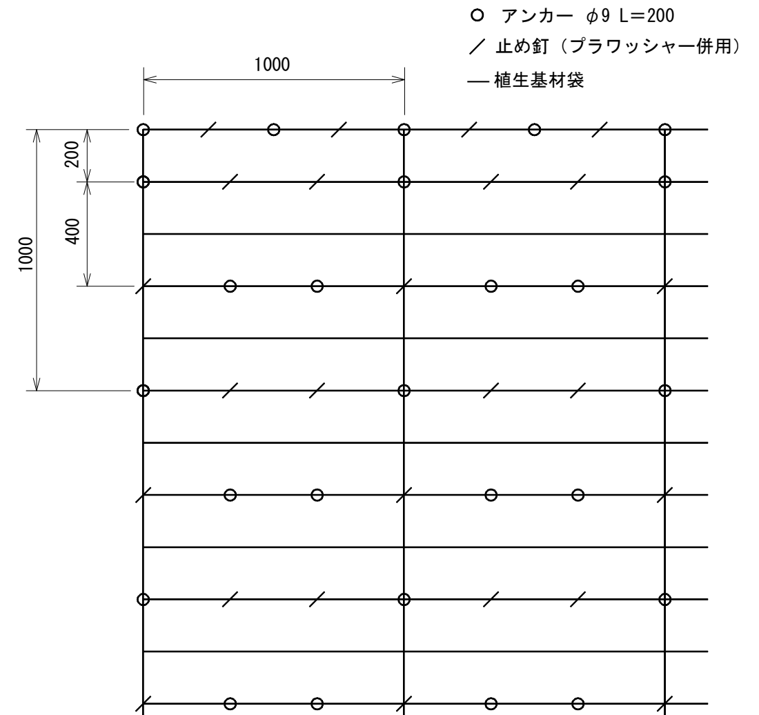
標準展開図
