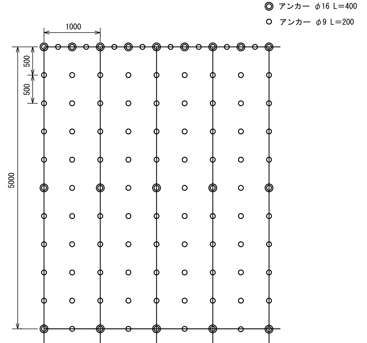
標準展開図
