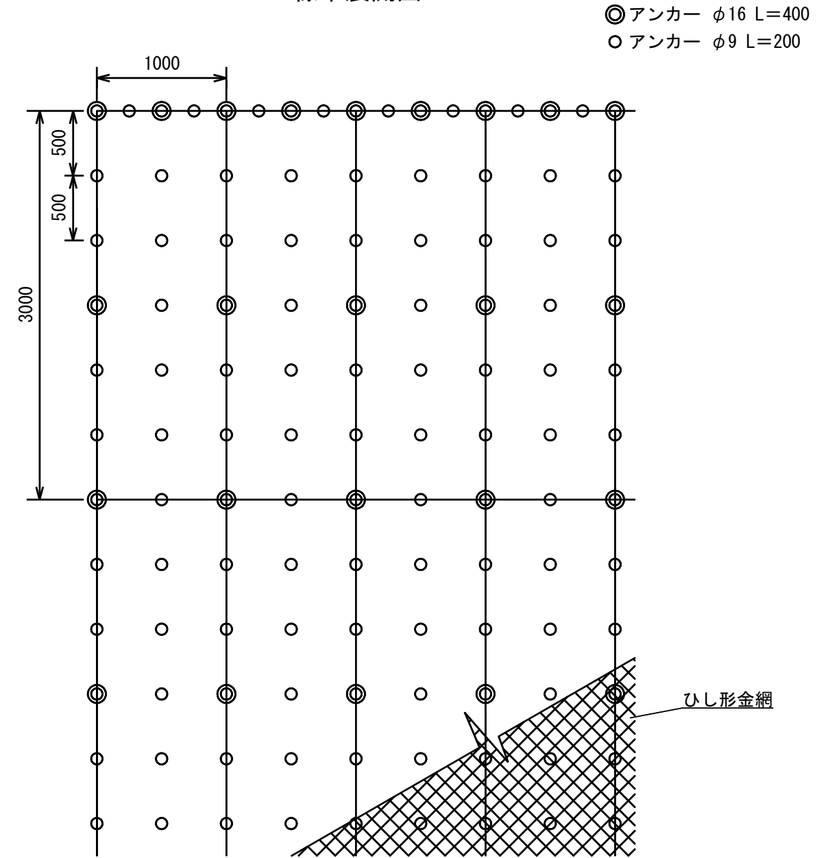
標準展開図
