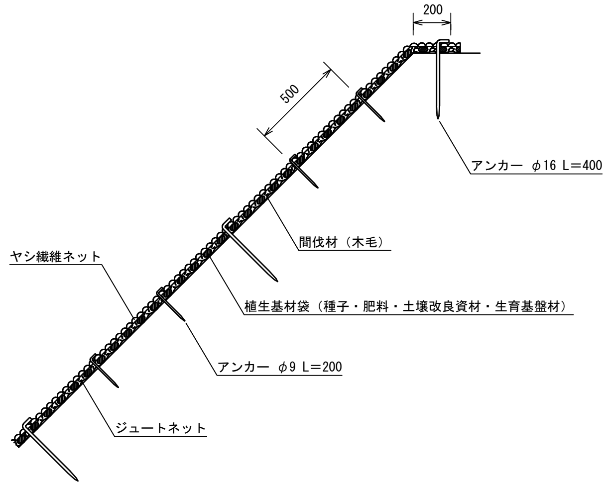
標準断面図
