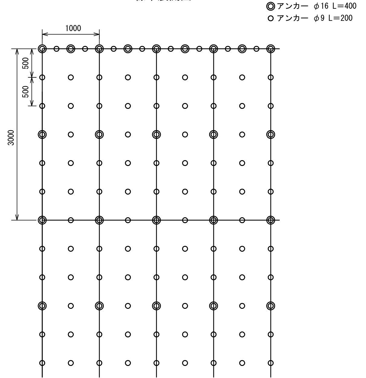
標準展開図
