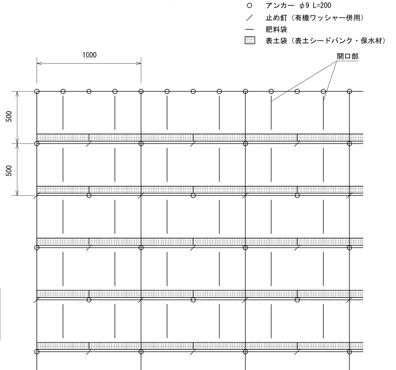
標準展開図
